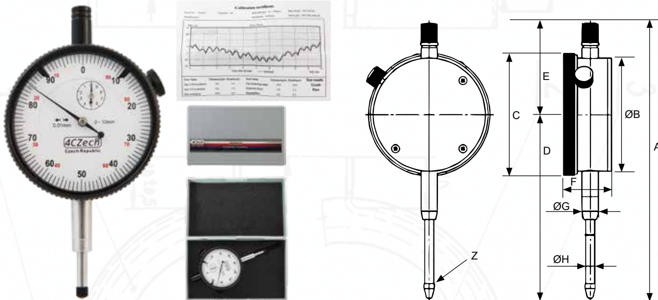
Úchylkoměr číselníkový (indikátor) ČSN EN ISO 46325 (ČSN 25 1811, 25 1816)
